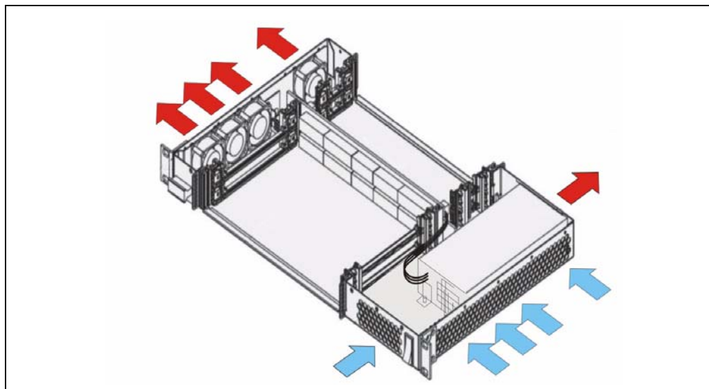
Figure 4: Entwärmung
