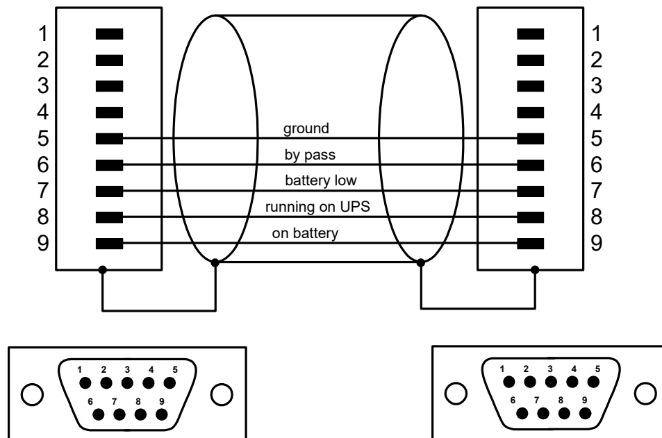
SUB D 9 Mâle / Male
