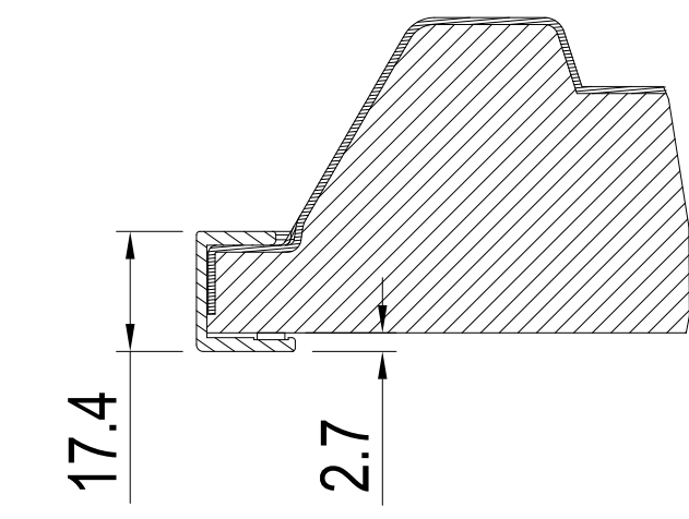
SECTION A-A SCALE 4:1
