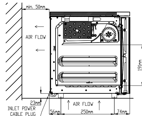
VISTA LATERALE SEZIONE B-B SIDE VIEW B-B SECTION
